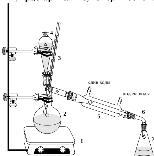
Рис. 1. Схема установки для проведения этерификации для получения эфира с температурой кипения ниже 100^{\circ}\text{C} .
